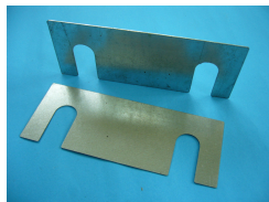
แผ่นขิมราง 5K
