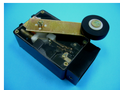
TOSHIBA LIMIT SW. QLU-2, QLU4
