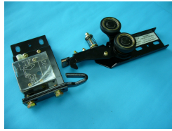
MITSUBISHI G01 DOOR LOCK - LEFT
